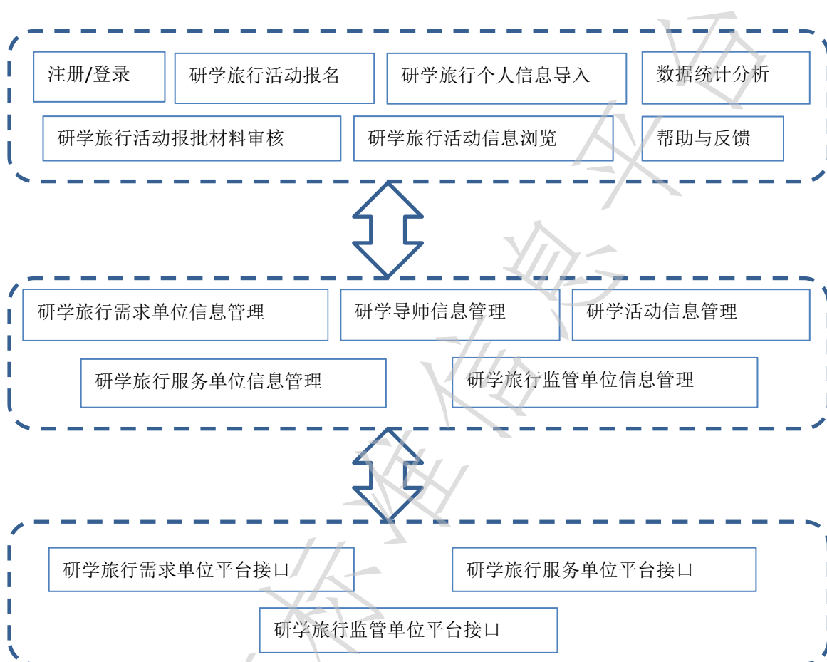
图 1 研学旅行信息管理平台软件结构
