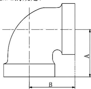
图A.2 异径弯头型式尺寸示意图
