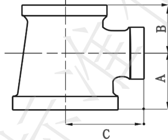
图A.3 侧大异径三通型式尺寸示意图
