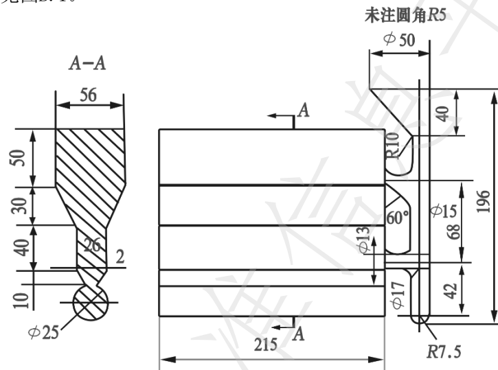
图B.1 球墨铸铁试块尺寸示意图
