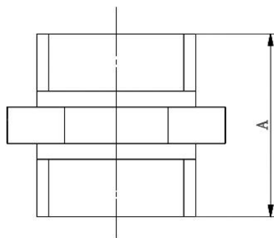
图A.7 活接头型式尺寸示意图
