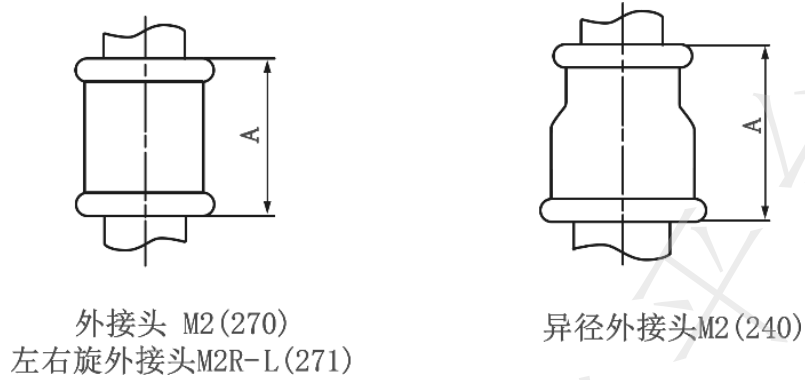
图A.6 外接头型式尺寸示意图
