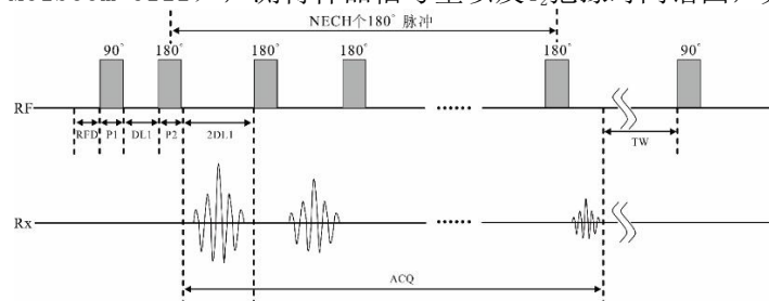
图1 硬脉冲 CPMG 序列图
