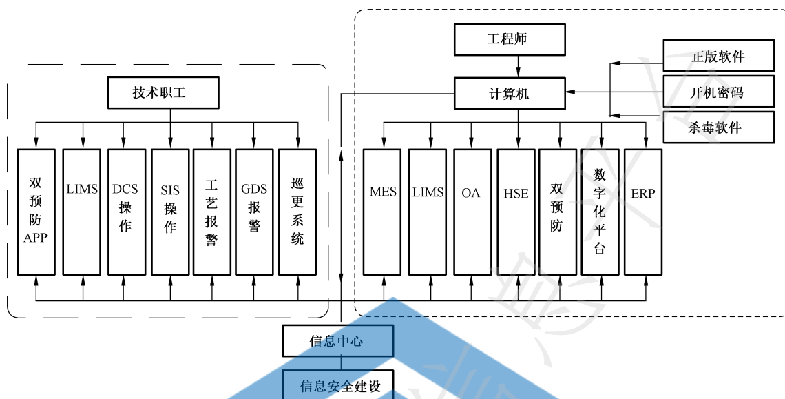
图6 车间信息化建设信息集成模型
