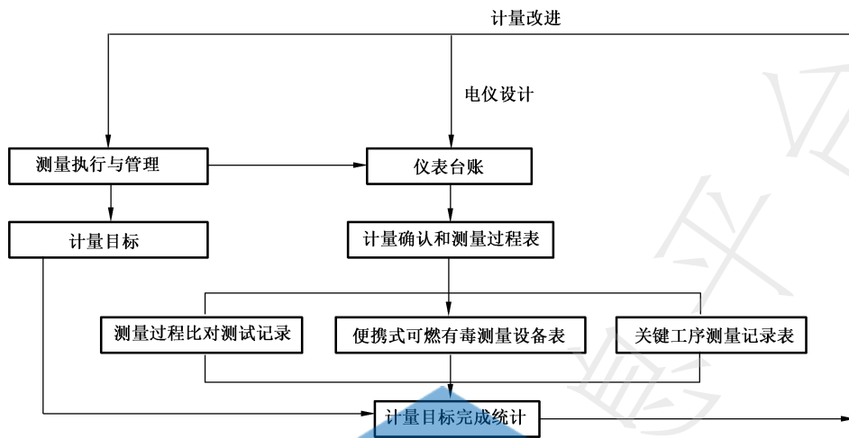
图 7 车间计量仪表管理信息集成模型
