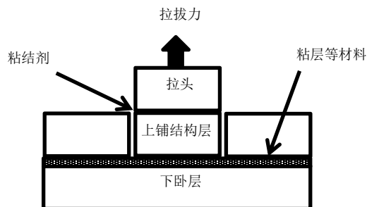
图 B.3 与下卧层的粘结强度试验时拉头粘结示意图
