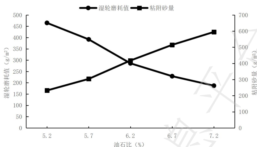
图 A.4 最佳油石比确定曲线
