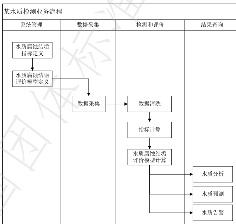
图 B. 2 业务流程设计参考图
