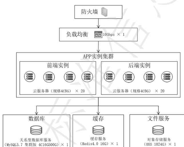
图 B.6 部署架构设计参考图
