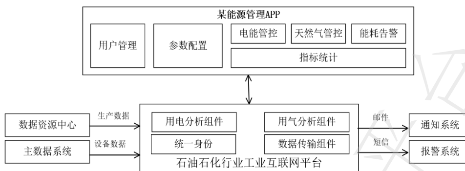
图 B.5 集成架构设计参考图
