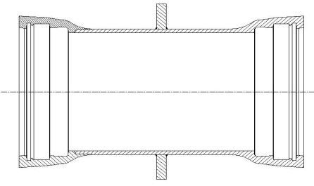
图 8 双承穿墙直管示意图
