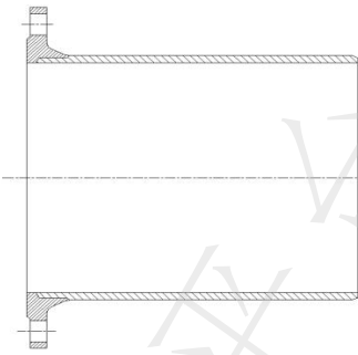
图 2 盘插直管示意图
