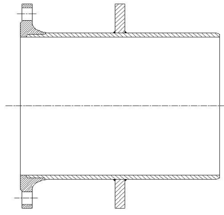
图 6 盘插穿墙直管示意图
