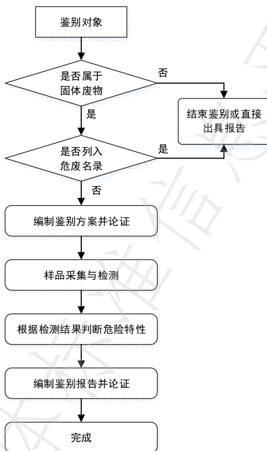
图1 固体废物危险特性鉴别工作流程图
