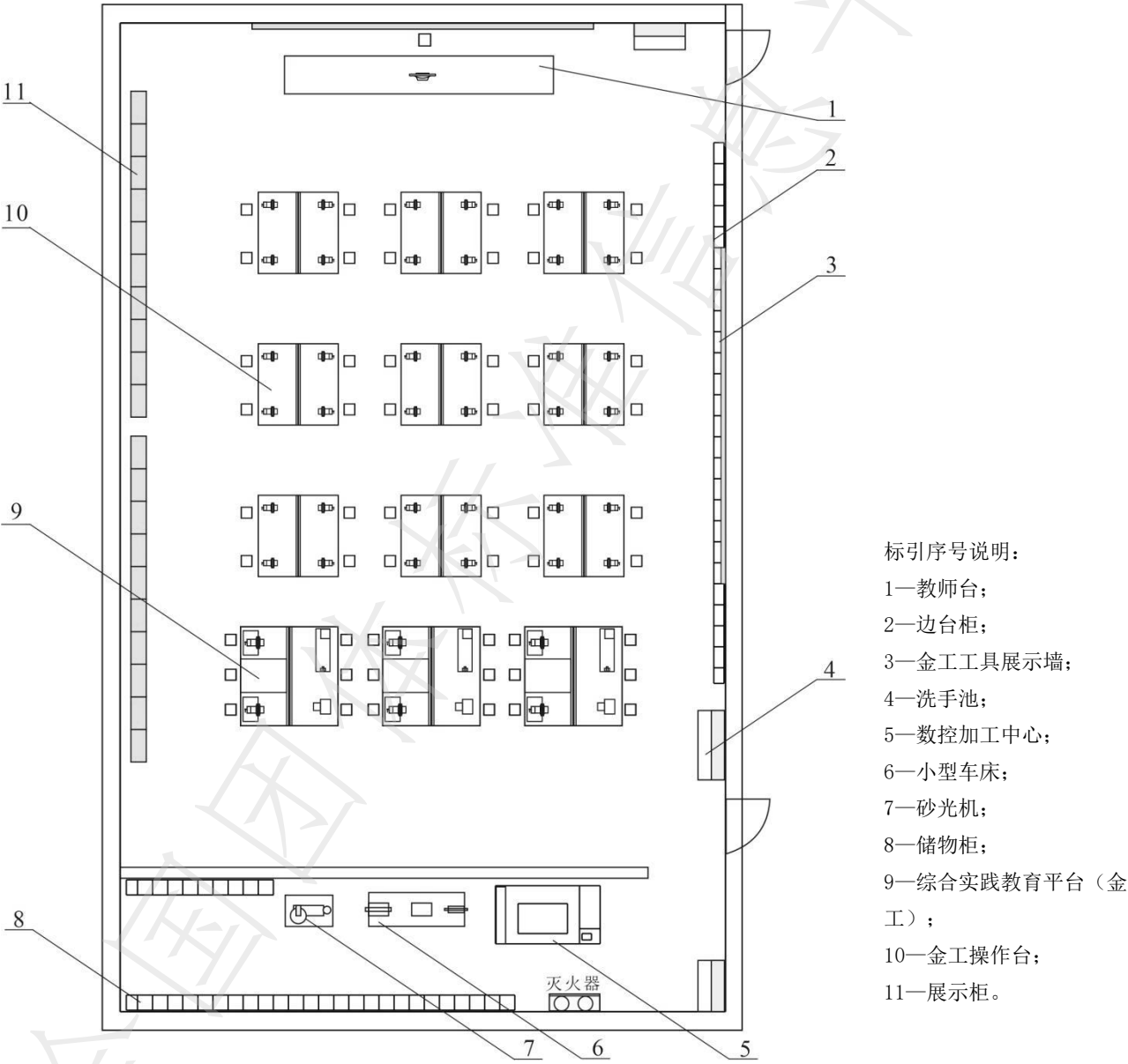
图 A.1 金工教室布置示意图（一）
