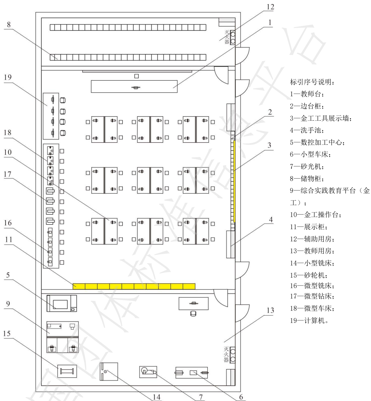
图 A.2 金工教室布置示意图（二）
