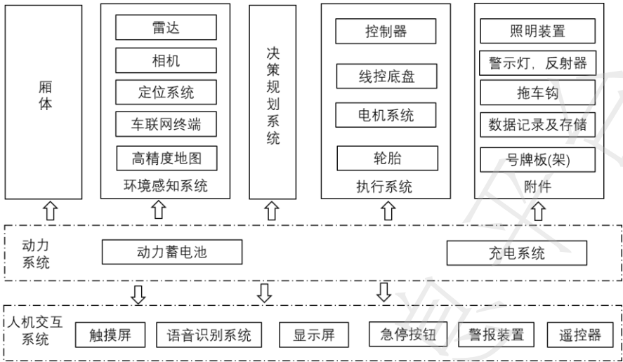
图1 无人驾驶配送装备结构示意图
