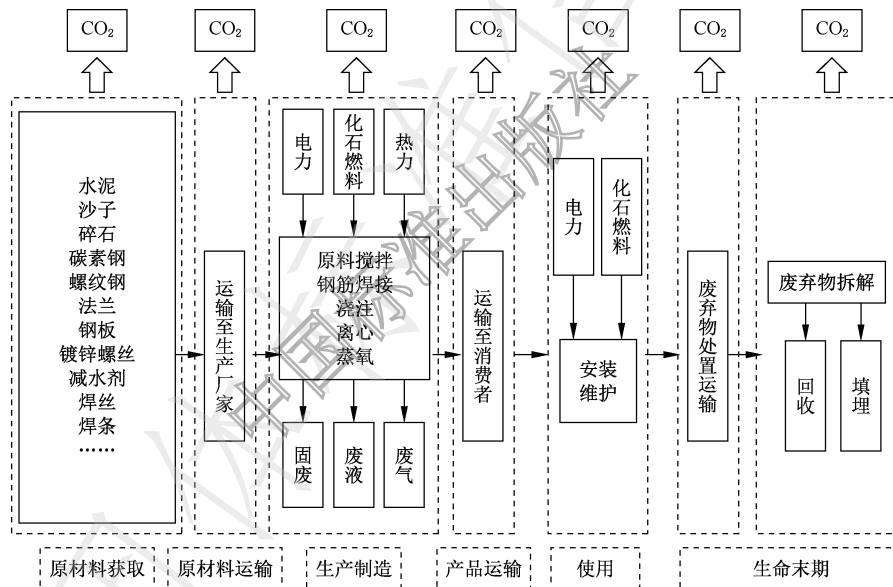
图1 混凝土电杆产品全生命周期系统边界示意图
