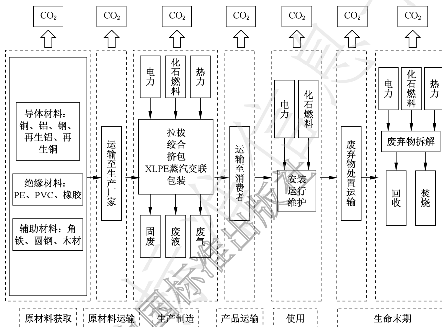
图 1 绝缘类导线产品全生命周期系统边界示意图
