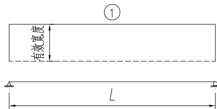
图3 简支梁计算图示
