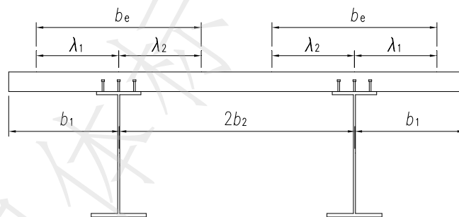
图 1 组合梁截面示意（未设承托）
