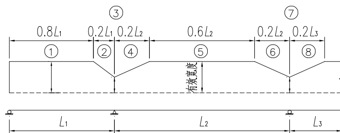
图4 连续梁计算图示
