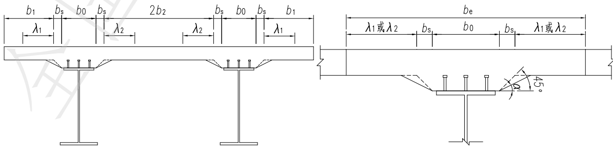
图 2 组合梁截面示意（设置承托）
