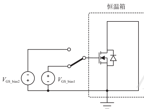
图1 高温栅偏试验电路参考
