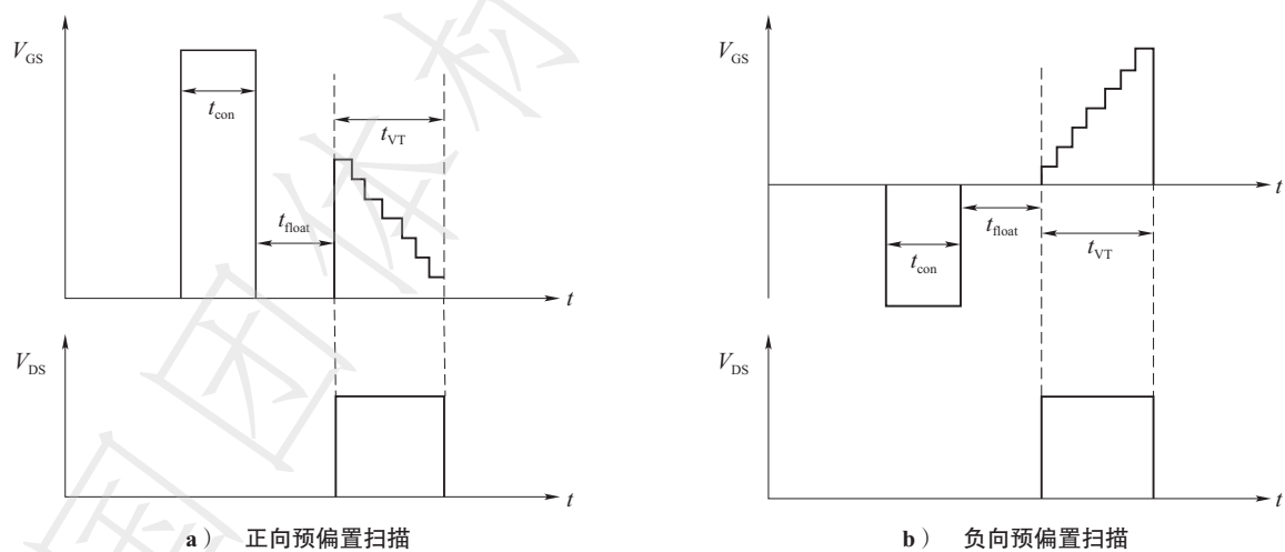
图3 双电压源扫描法测试时序
