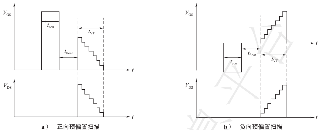
图5 单电压源扫描法测试时序
