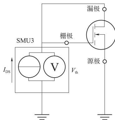
图6 电流源法测试电路
