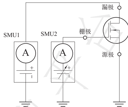
图2 双电压源扫描法测试电路
