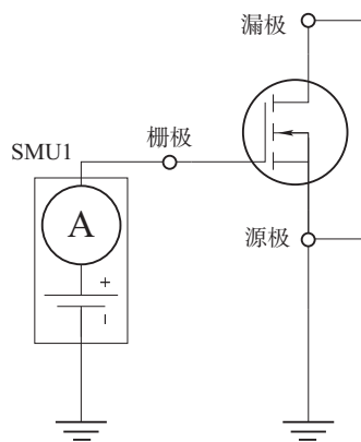
图1 栅极预偏置电路
