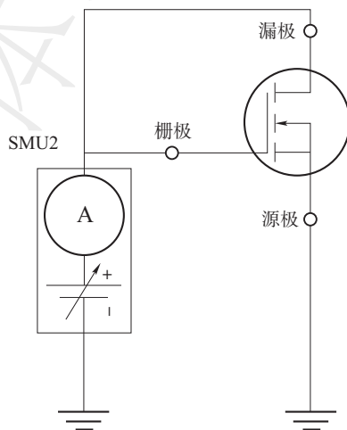
图4 单电压源扫描法测试电路
