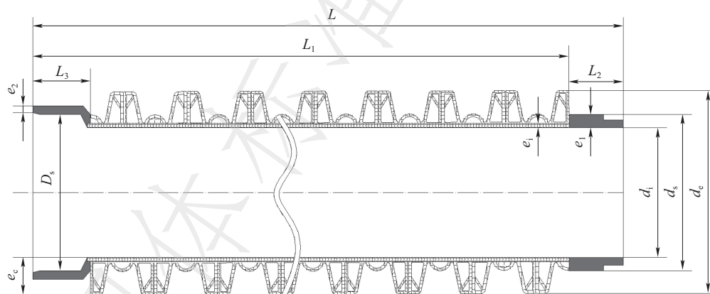
图2 管材结构示意图
