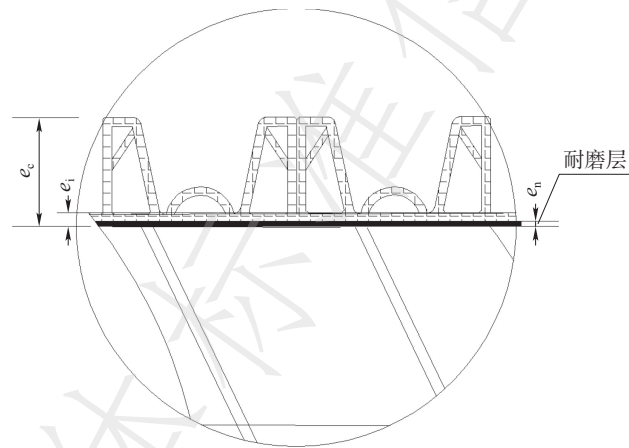
图1 管材结构示意图
