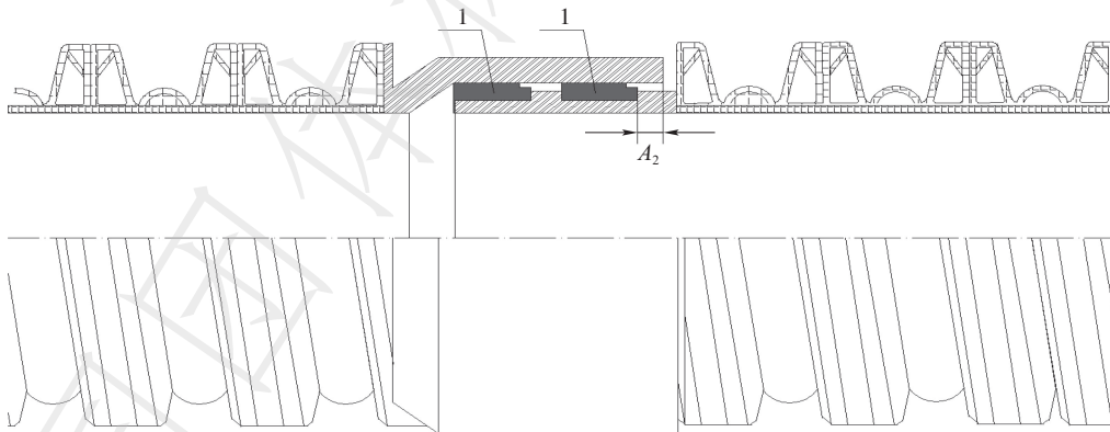
图 A.1 电热熔+密封橡胶圈连接示意图
