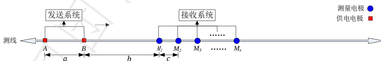
图2 通用偶极-偶极装置示意图
