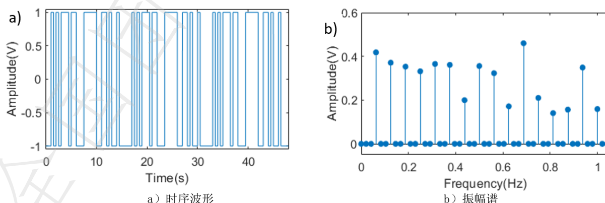
图 E.1 5 阶扩频波的时序波形和振幅谱
