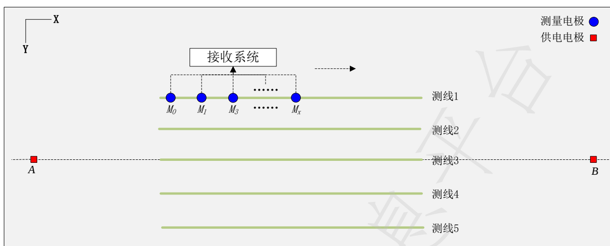
图1 中间梯度装置示意图
