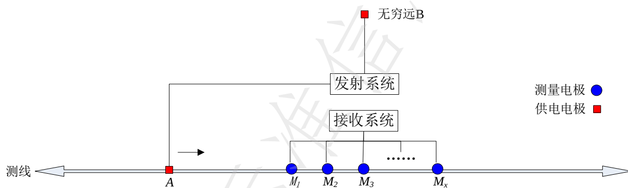
图3 通用三极装置示意图
