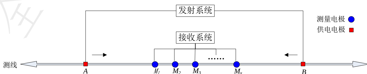
图4 通用四极装置示意图
