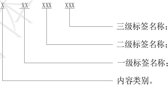
图 1 代码结构图
