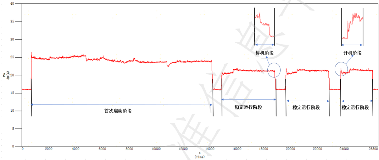
图 A.1 压缩式制冷器具运行工况时域示意图
