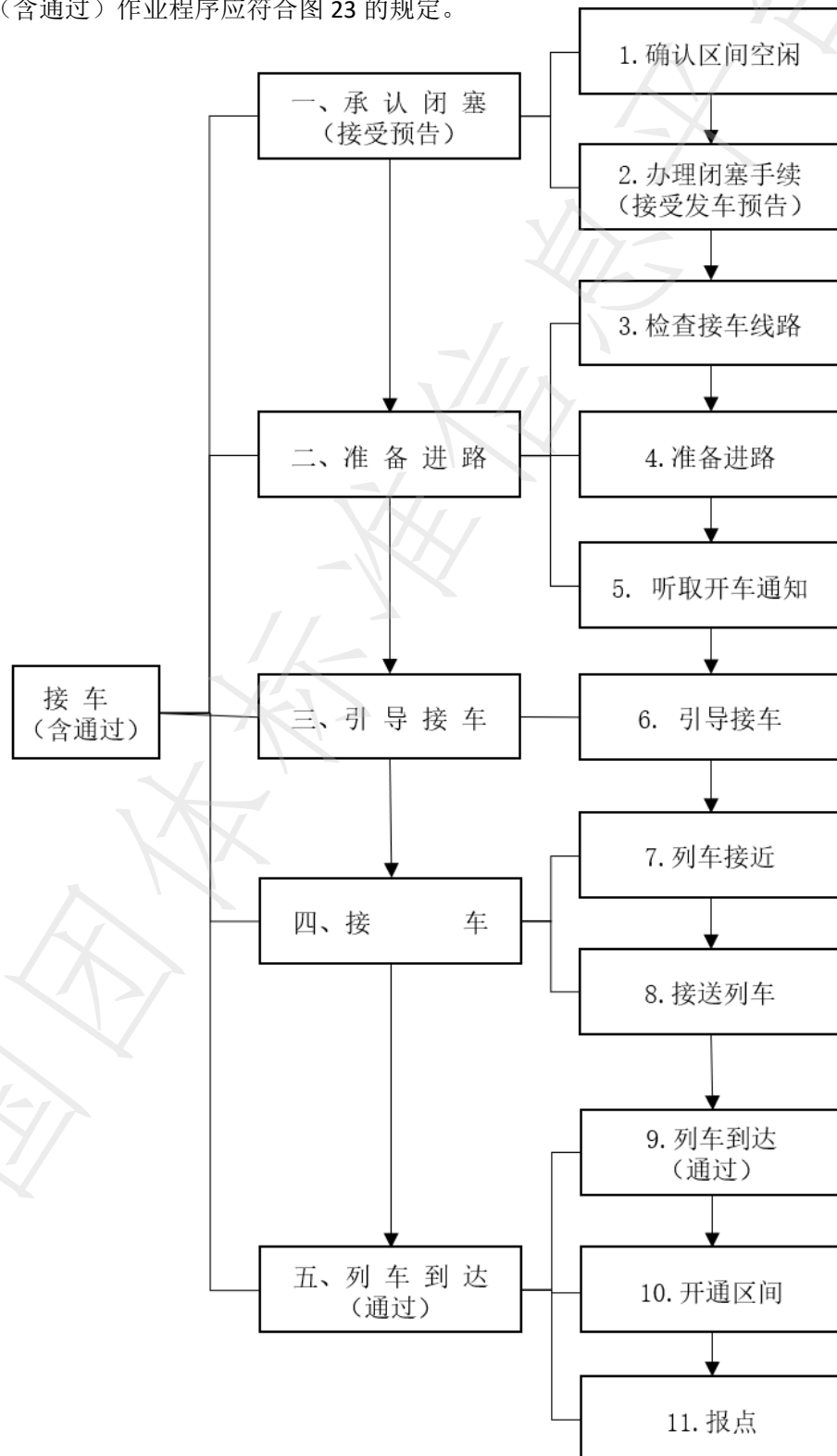
图 23 接车（含通过）作业程序
