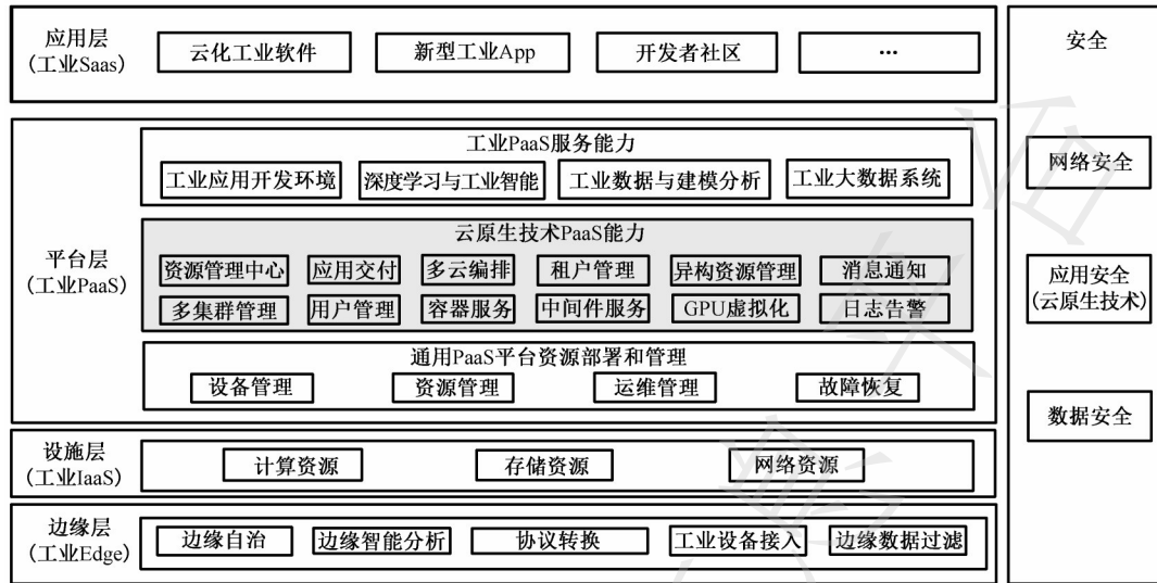
图1 钢铁行业工业互联网云原生技术参考架构
