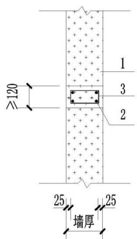
快硬改性轻质石膏墙墙体高度超过6m时，宜在墙体半高处设置暗梁
