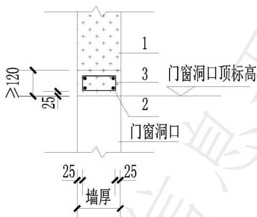
图 4.3.4 洞口处暗梁
