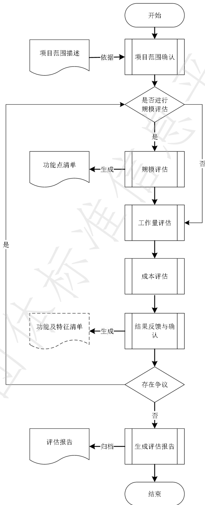
图 1 软件造价评估总体流程
