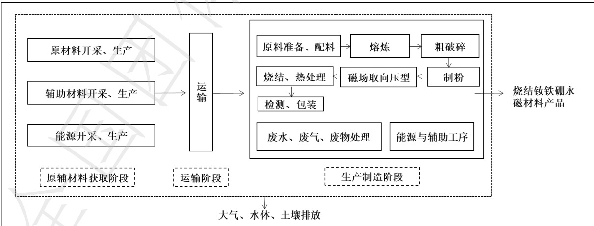
图 1 系统边界图
