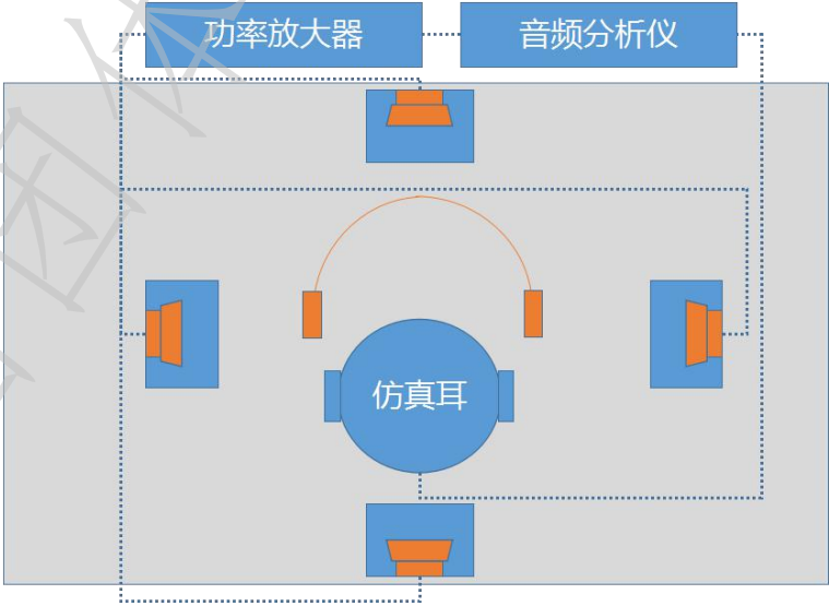
图1 测试示意图1
