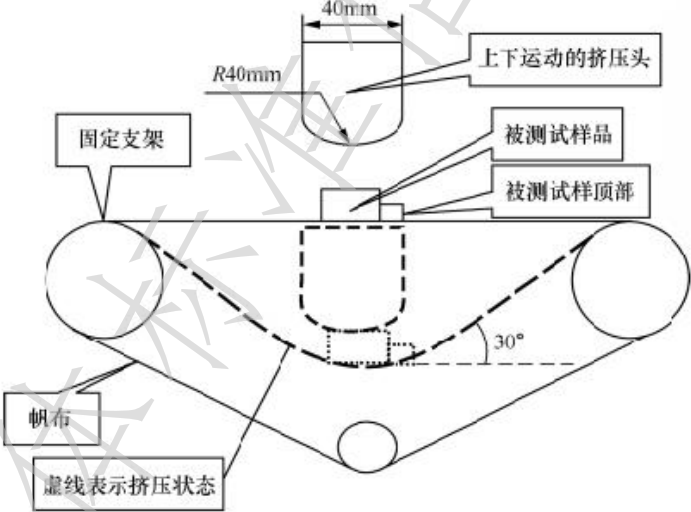
图1 试验示意图
