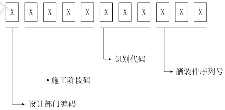
图B. 4 电气舾装件命名示意图
