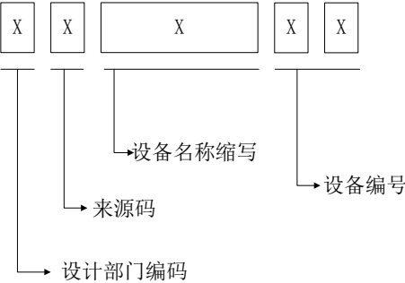
图B.7 设备命名示意图
