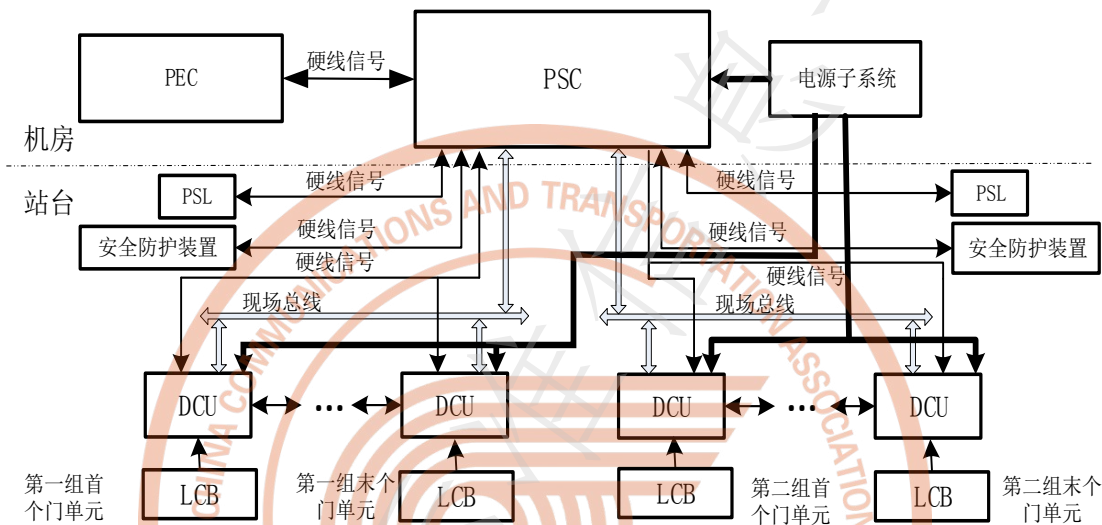
图5 电气系统组成示意
