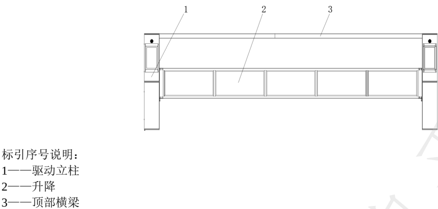
图9 升降式站台门结构试验样机示意
