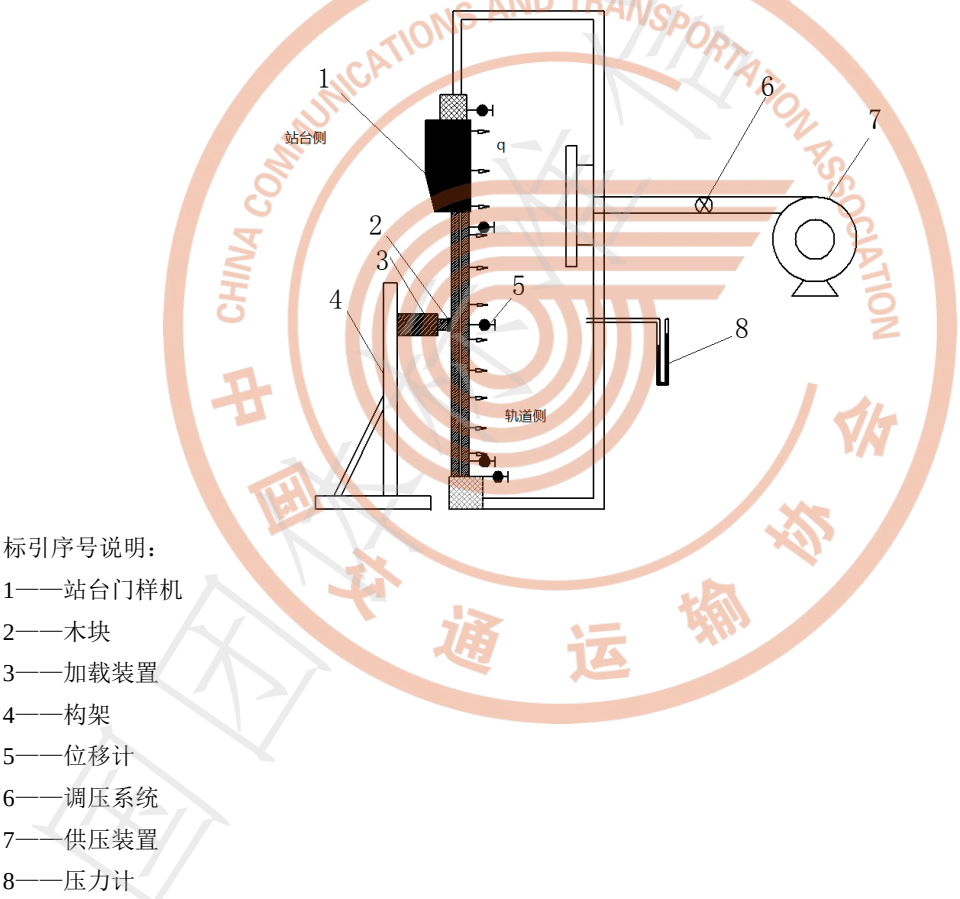
图19 全高站台门风压载荷试验和乘客挤压载荷联合试验装置
