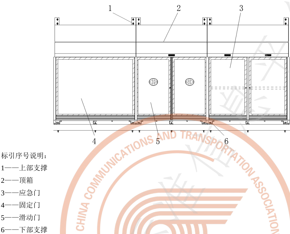
图3 全高站台门机械结构示意
