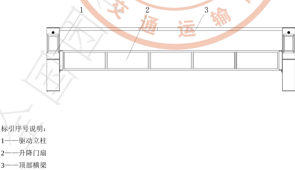
图4 升降式站台门机械结构示意
