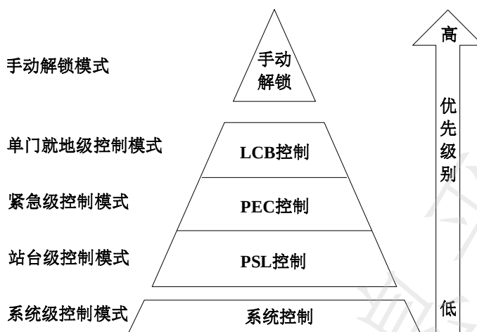
图6 站台门系统控制模式示意
