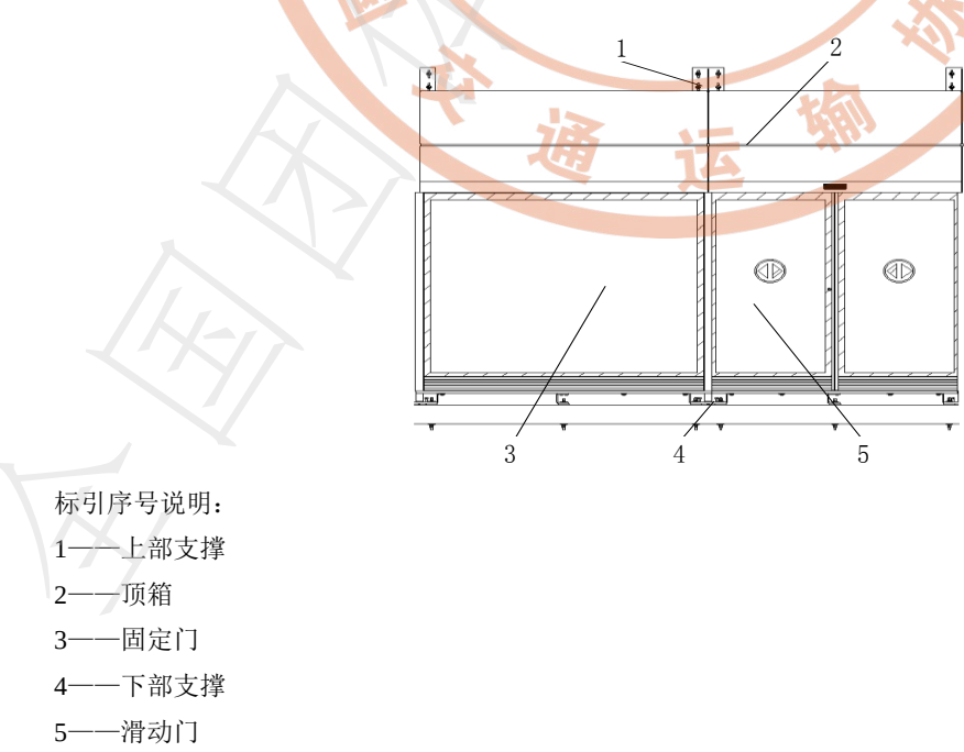
图8 全高站台门结构试验样机示意
