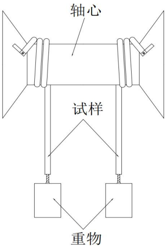
图 12 低温卷绕
