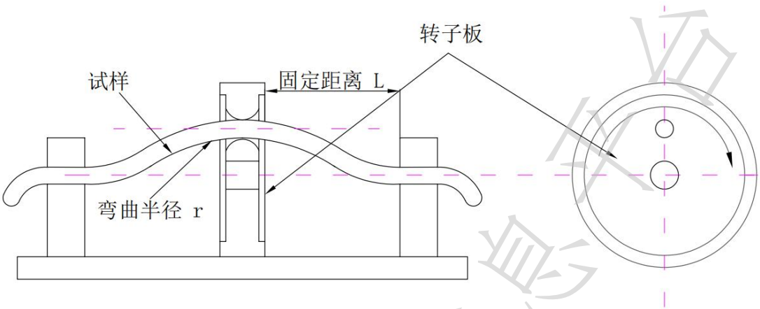
图 2 弯折及旋转示意图
