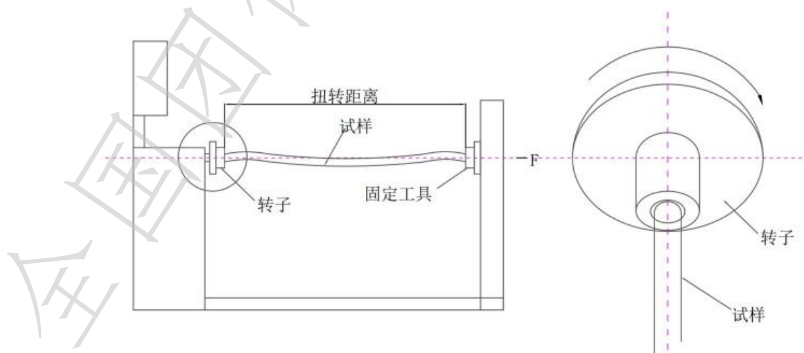
图 5 2D 扭转示意图
