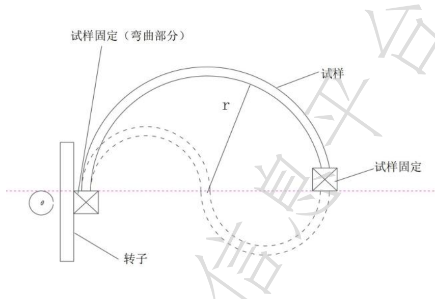
图 6 曲线扭转示意图
