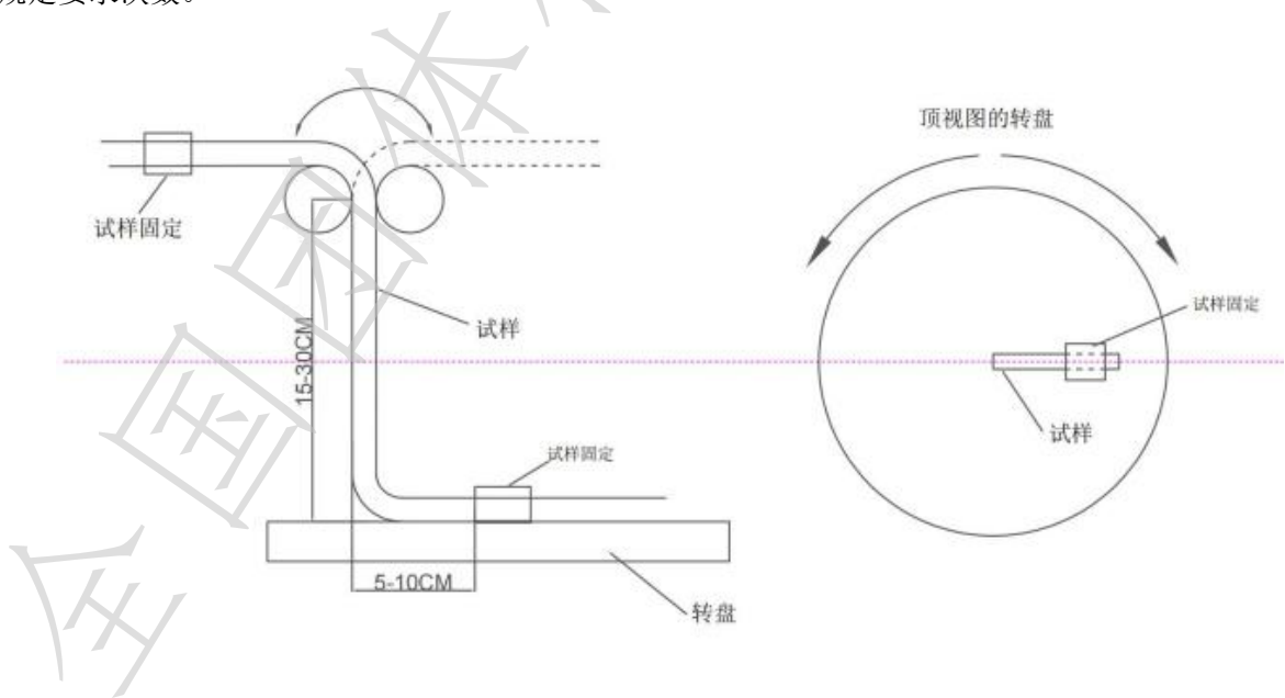
图 7 3D 扭转示意图
