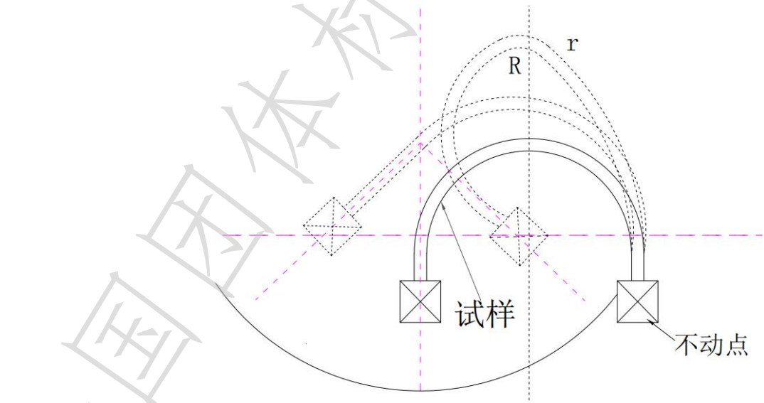
图 3 快速弯折示意图
