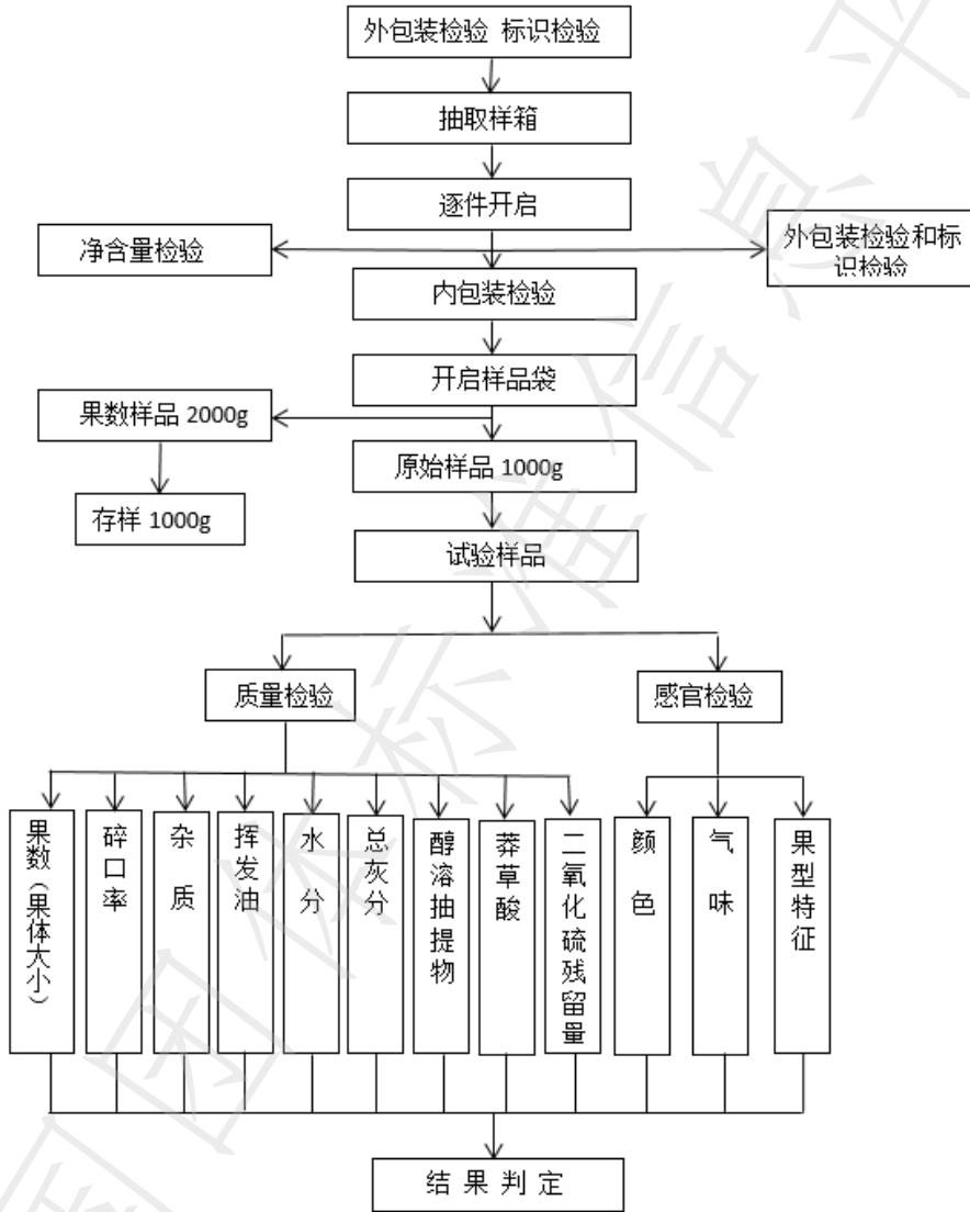
图A.1 产品检验流程图
