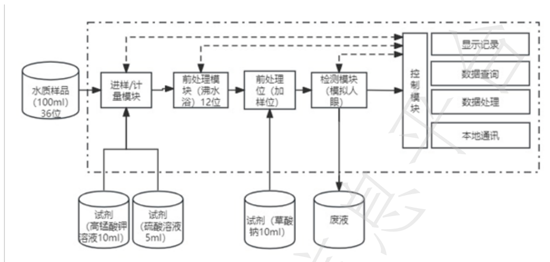
图A.1 高锰酸盐指数自动分析仪结构图
