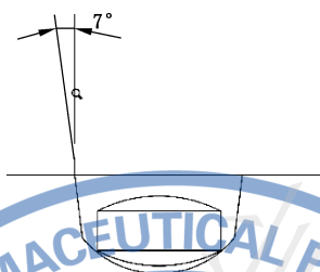
图 5 冷成型泡眼示例
