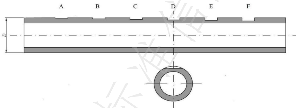
图2 02型标定管上人工缺陷的形状及位置示意图
