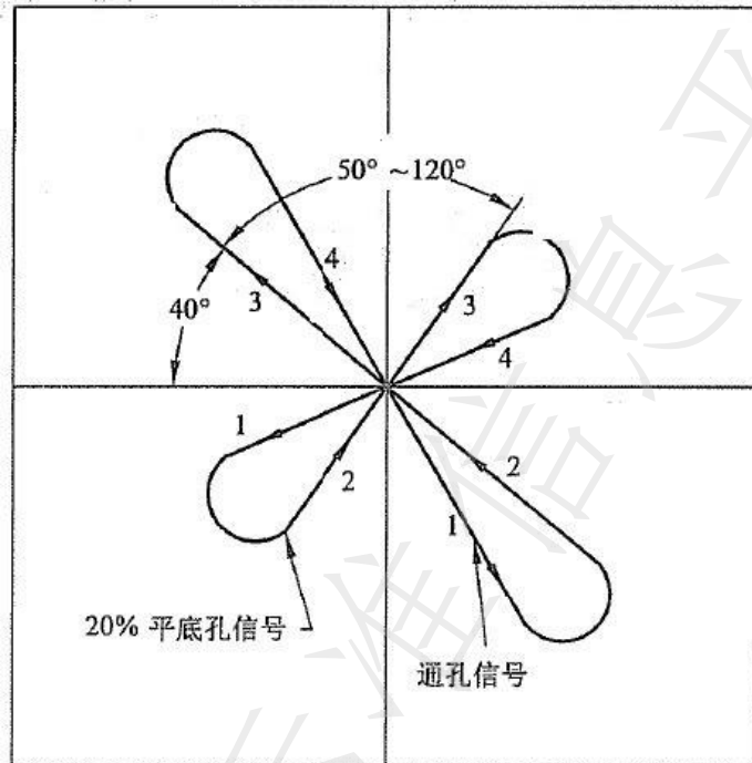
图 3 差分通道经过正确调整的典型涡流信号阻抗平面图
