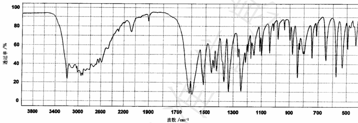
图A.1 L-酪氨酸标准品红外光谱图
