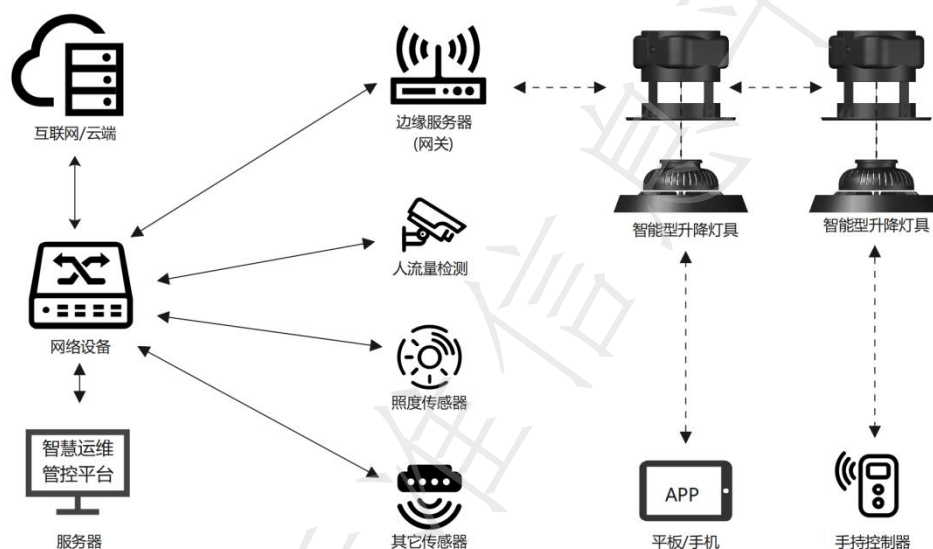
图1 升降灯具的系统组成与工作原理示意图
