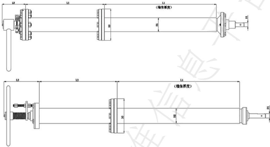
图 A. 8 穿墙/地式操作台
