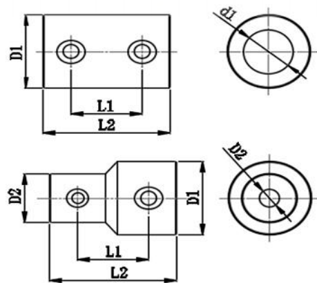
图 A. 20 连接套
