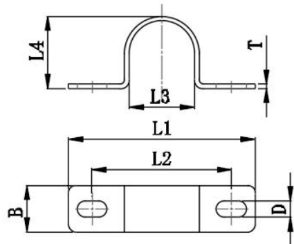
图 A. 23 不锈钢型轴卡
