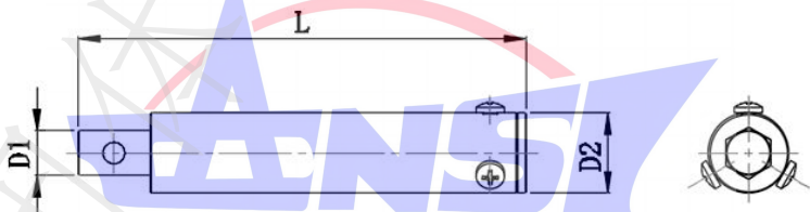
图 A. 21 伸缩杆
