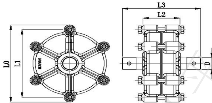
图 A. 19 扭矩倍增器
