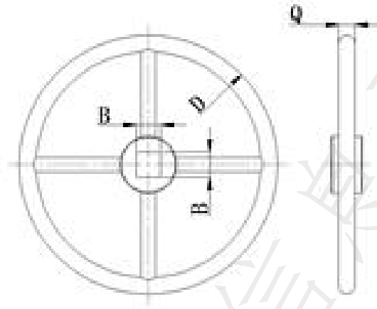
图 A.25 不锈钢手轮
