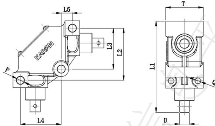
图 A. 16 L 型转向器
