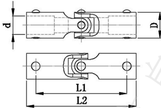
图 A. 10 两节型万向节
