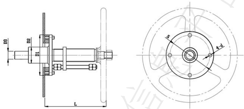
图 A. 7 穿舱型操作台
