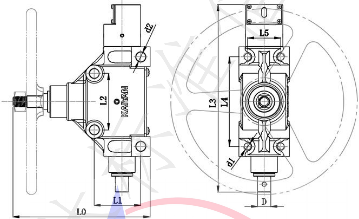
图 A.3 双头 T 型操作台 表 A.3 双头 T 型操作台型号和尺寸
