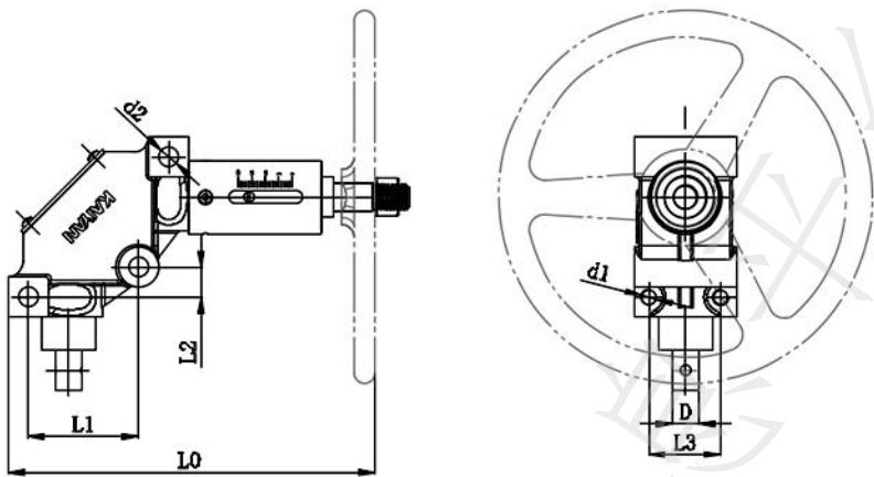
图 A. 4 L 型操作台
