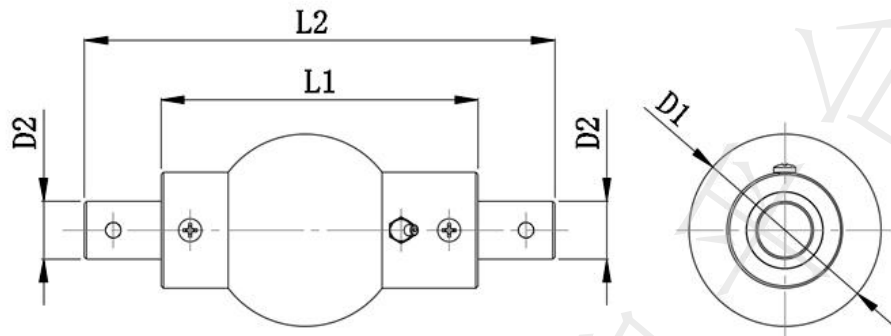
图 A. 13 球型贯穿件
