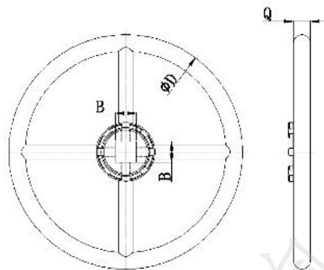
图 A. 26 不锈钢离合式手轮
