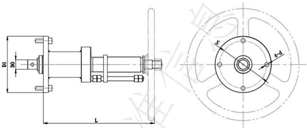
图 A. 1 立式操作台
