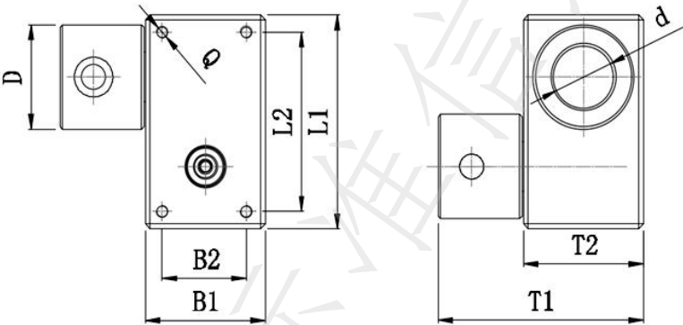
图 A. 18 X 型转换器
