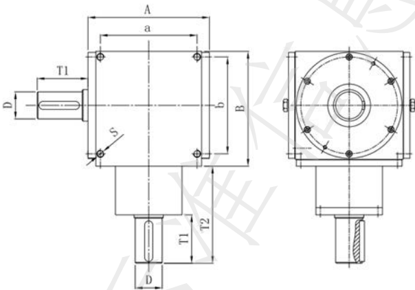
图 A. 15 F 型转向器
