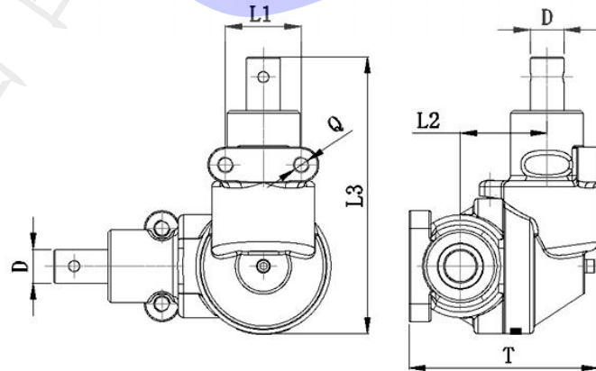
图 A. 17 C 型转换器
