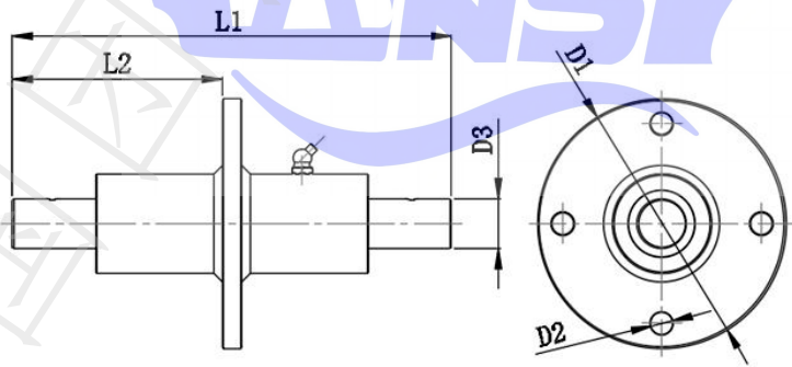
图 A. 14 法兰型贯穿件
