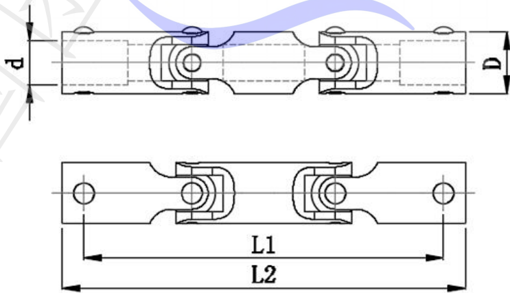
图 A. 11 三节型万向节
