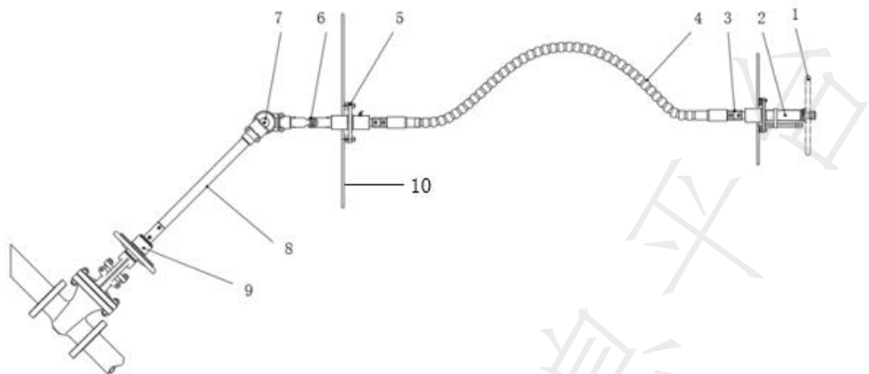
标引序号说明： 1——手轮； 2——立式操作台； 3——连接套； 4——柔性轴； 5——法兰型贯穿件； 6——万向节； 7——C型转向器； 8——刚性轴； 9——适配器 10——舱壁
