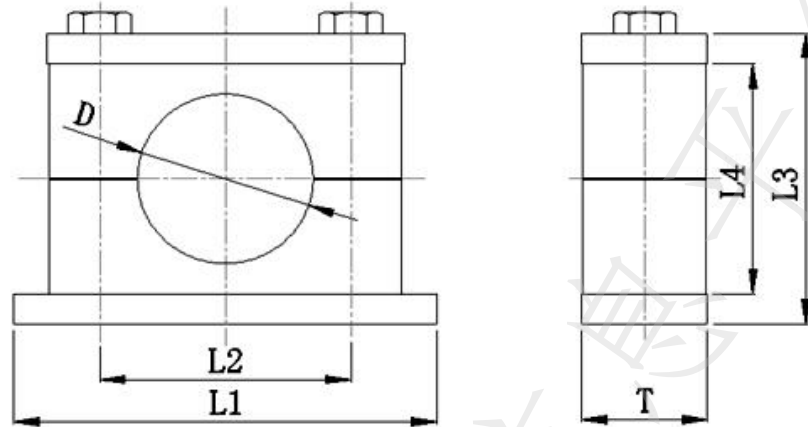
图 A. 22 塑料型轴卡
