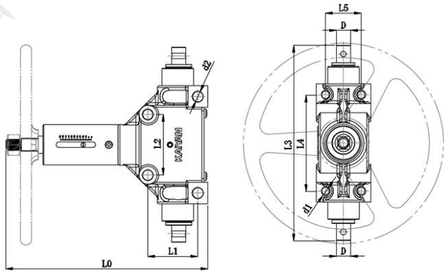
图 A. 2 单头 T 型操作台
