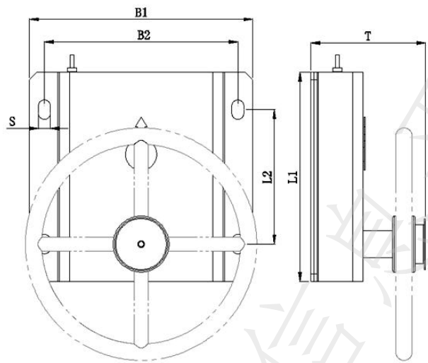
图 A. 9 绞盘式操作台
