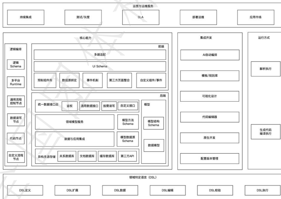
图 1 企业级低代码开发平台系统架构
