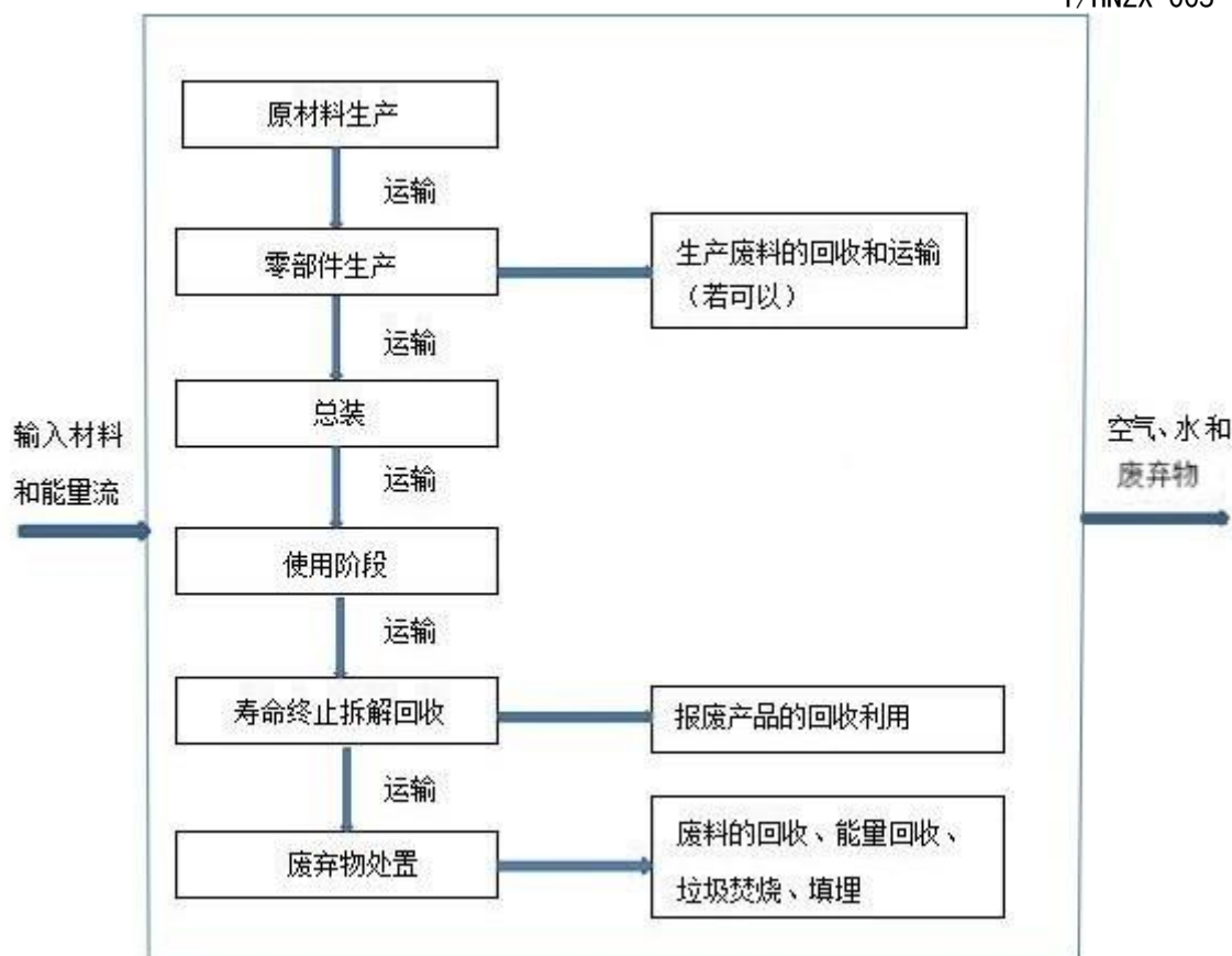
图 B.1 泵车耐磨弯管生命周期评价系统边界
