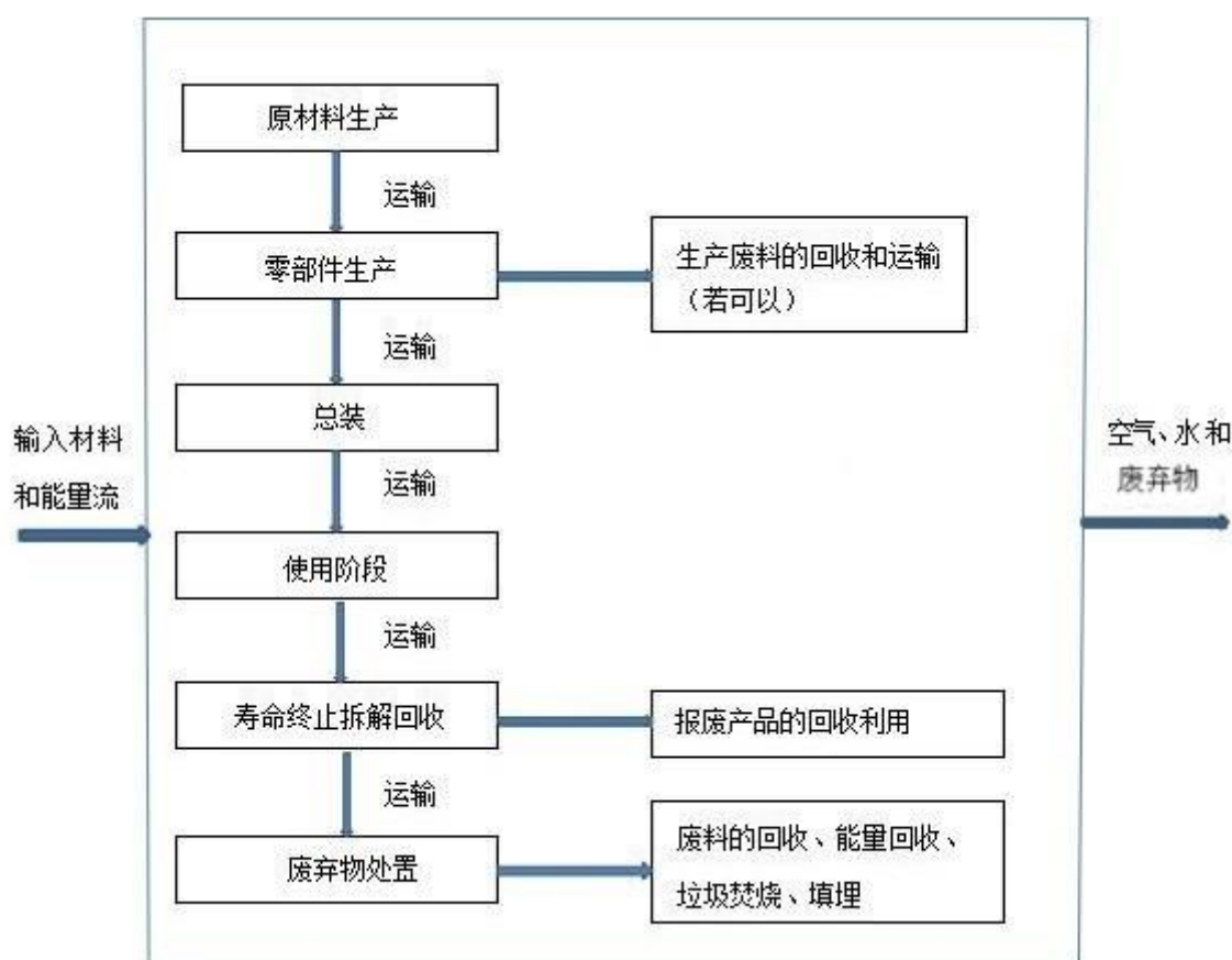
图 B.1 高锰钢耐磨件生命周期评价系统边界
