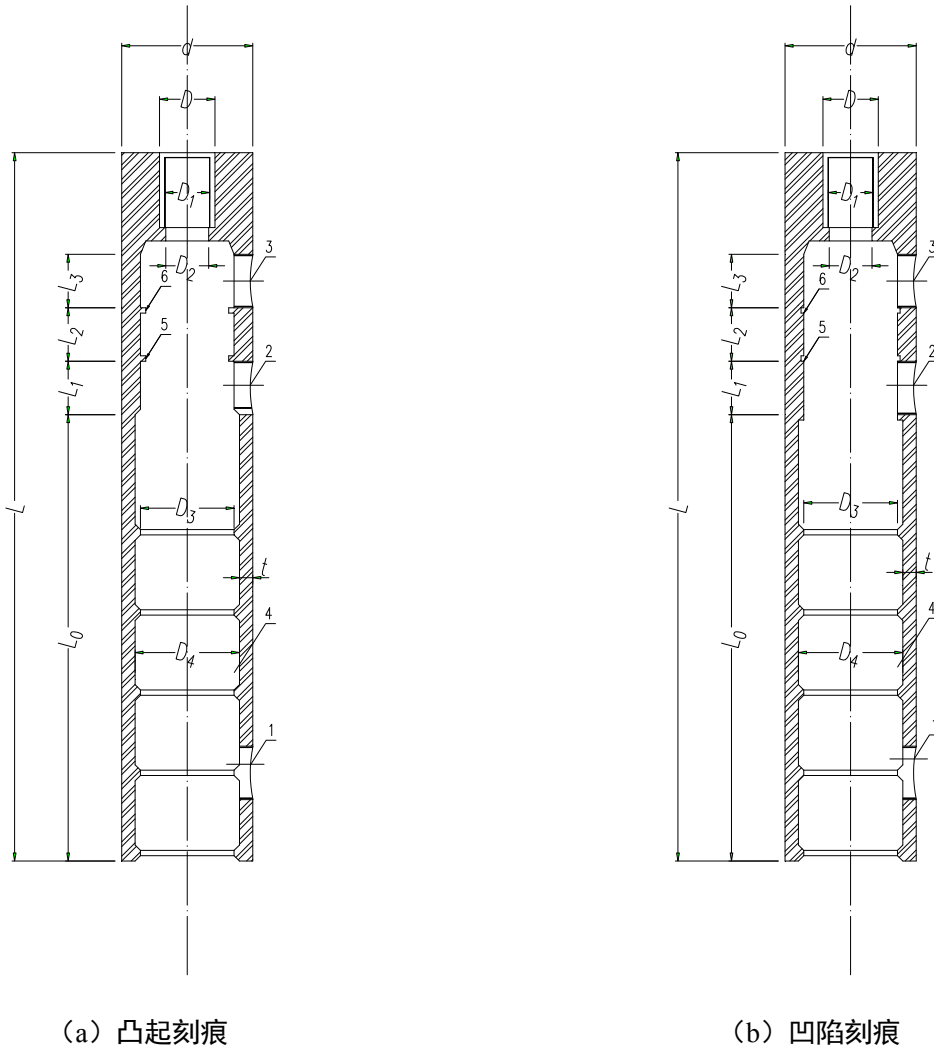
图 2.1.11 缺陷可检修型半灌浆套筒
