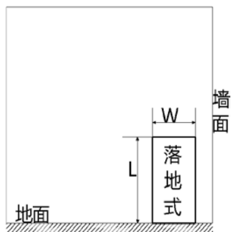
图A.6 分体落地式空调器室内机安装示意图
