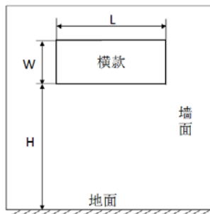
图 A.4 横款分体挂壁式空调器室内机安装示意图
